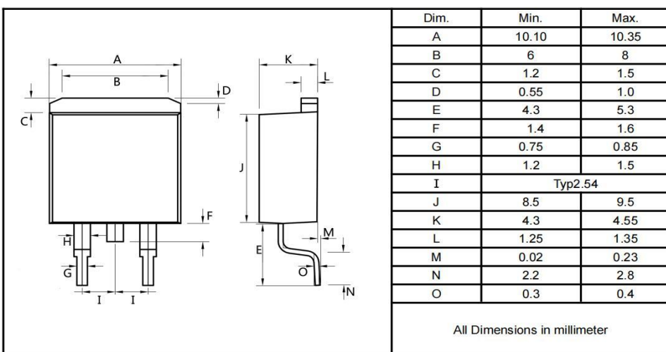
TO-263
