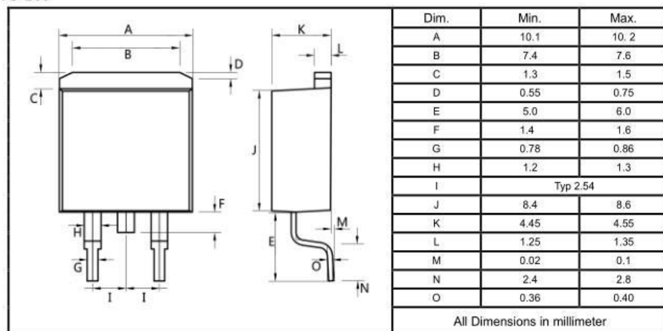
TO-263
