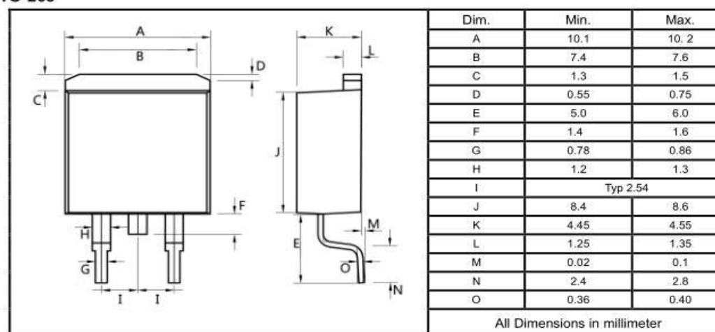
TO-263
